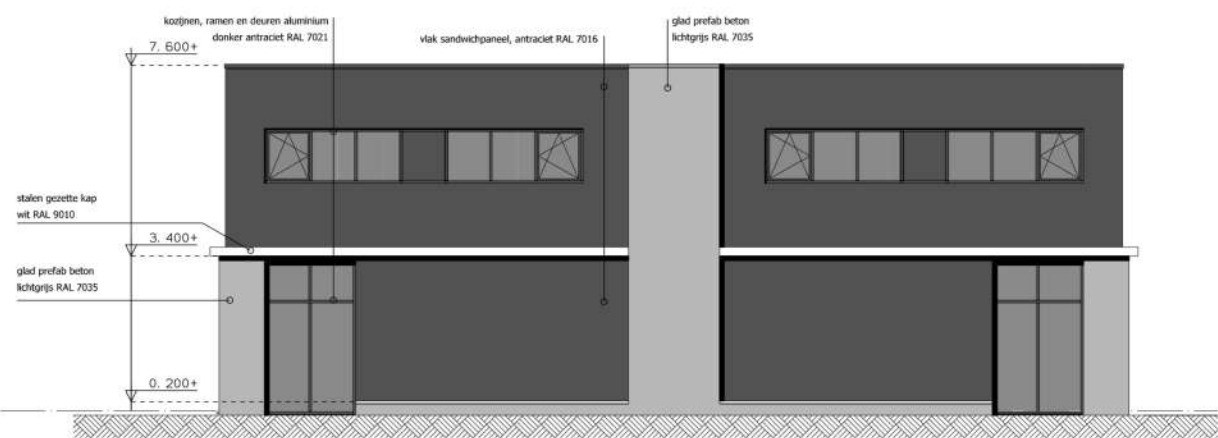
rechter zijgevel
